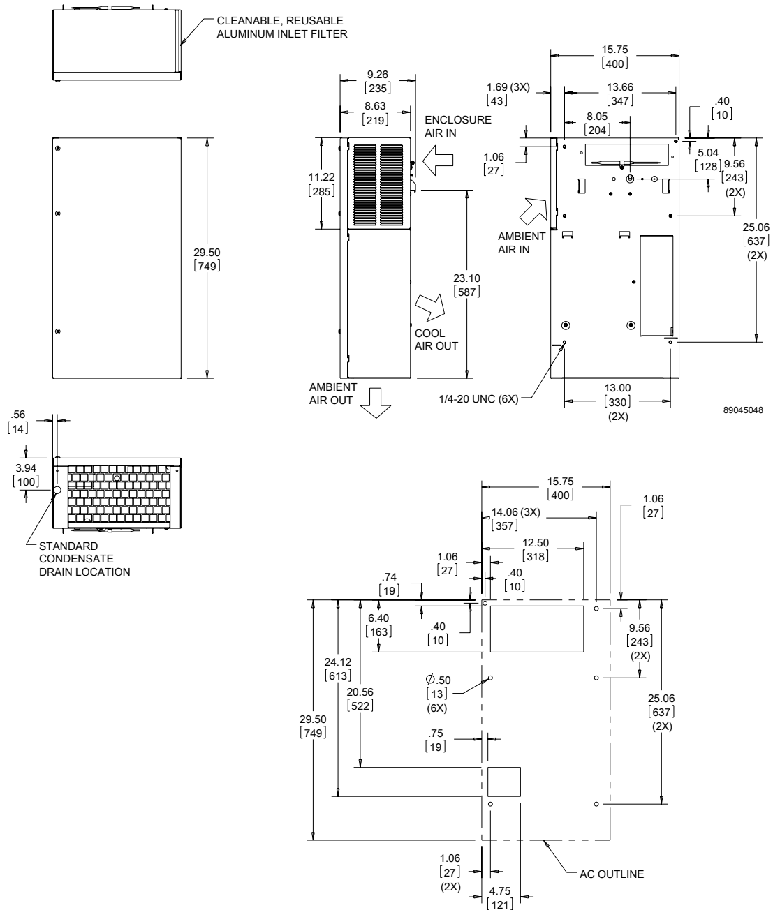
Cutout Dimensions
