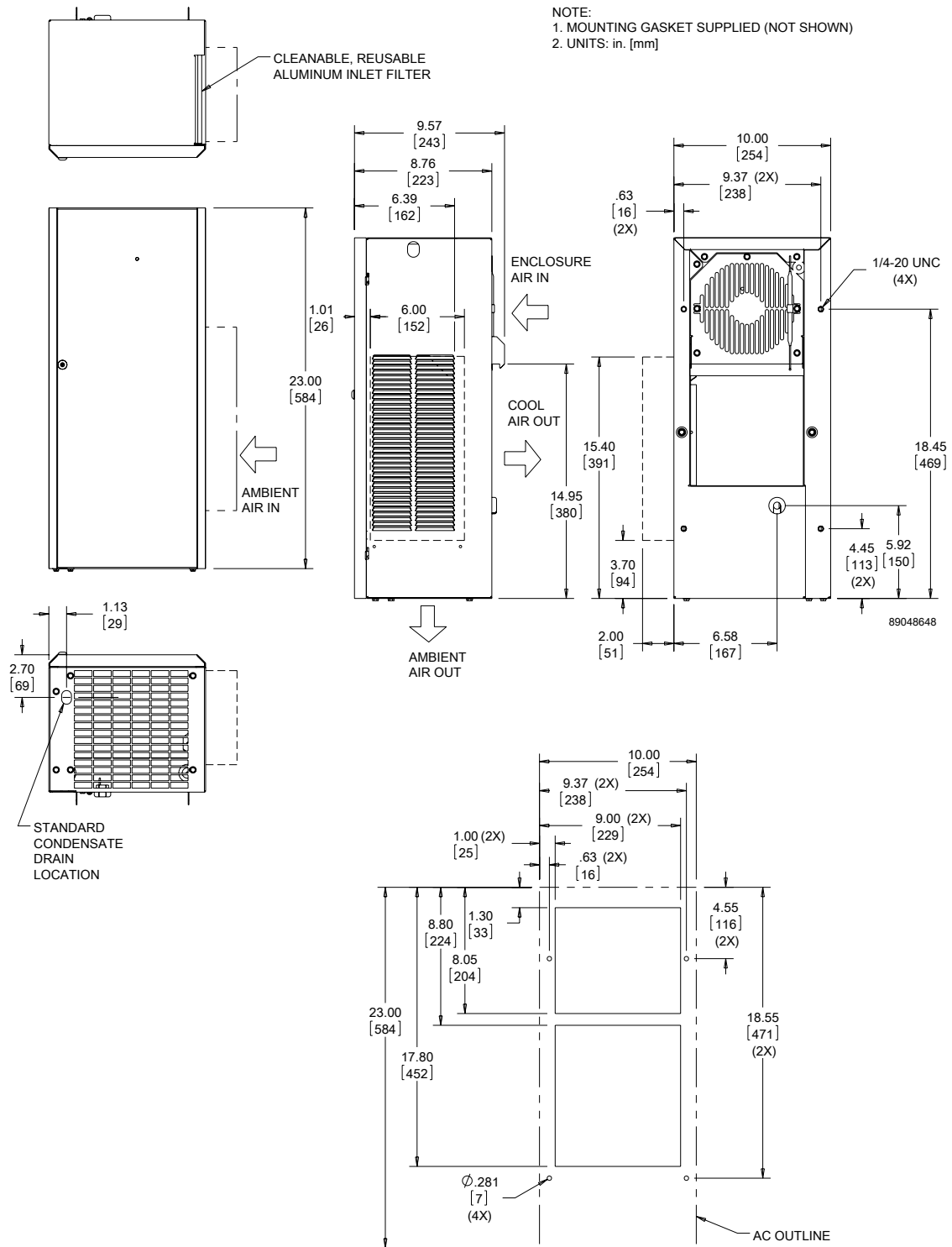
Cutout Dimensions
